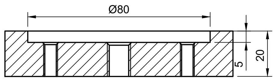
A-A (1:1)
